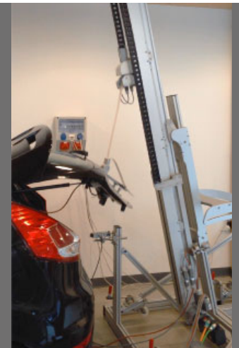
Heckklappe / back door
